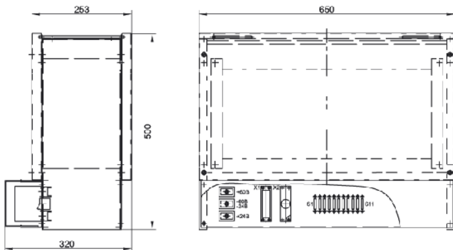
Габаритный чертеж блока резисторов
